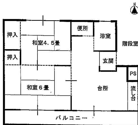
如意谷住宅 A棟104号
